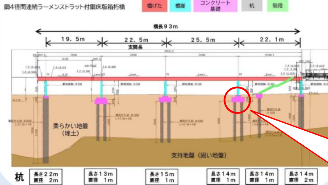
歩道橋構造図 (真横からみた図面)
